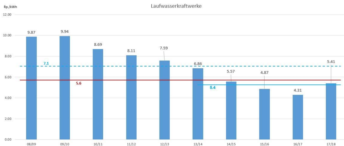
Abbildung 4: Historische Erlöse für Laufwasserkraftwerke / Berechnungen des ior/cf-HSG auf Basis EEX, EpexSpot; vollständige Gestehungskosten gemäss BFE 2018 [1c]; ohne Handel mit Herkunftsnachweisen.
